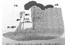
「谷根川の大釜」は、谷根川左岸の岩盤にできたくぼみで、深さは最大4.7m
